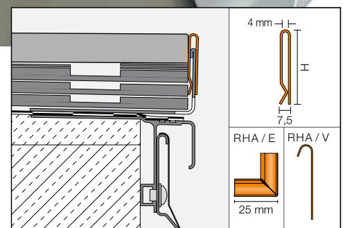
Schlüter®-BARA-RHA auf Schlüter®-BARA-RWL
